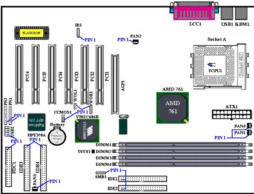
Figure 2-7. Tous les connecteurs et Switches de la KG7-Lite/KG7/KG7-RAID
