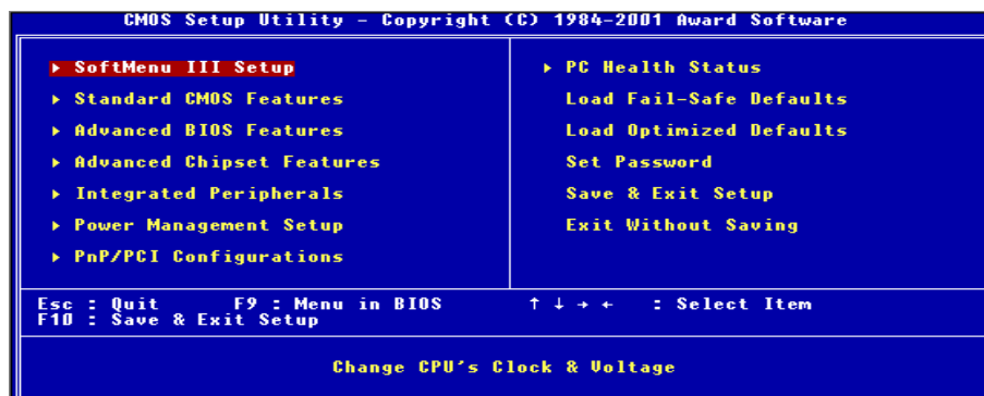
Figure 3-1. Utilitaire du CMOS Setup
