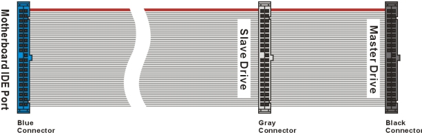
Figure 2-10. Schéma d'une nappe de connexion Ultra DMA 66
