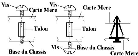
Figure 2-2. La manière de fixer la Carte Mère
