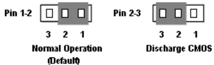
Figure 2-8. Positions du CCMOS1
