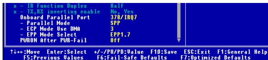
Figure 3-6B. Partie inférieure de l'Integrated Peripherals Menu
