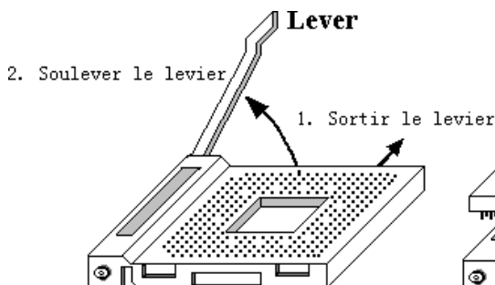
Schema 2-3. Socle A et son levier ouvert
