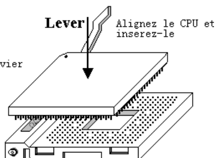
Schema 2-4. Installer le CPU dans le Socle A
